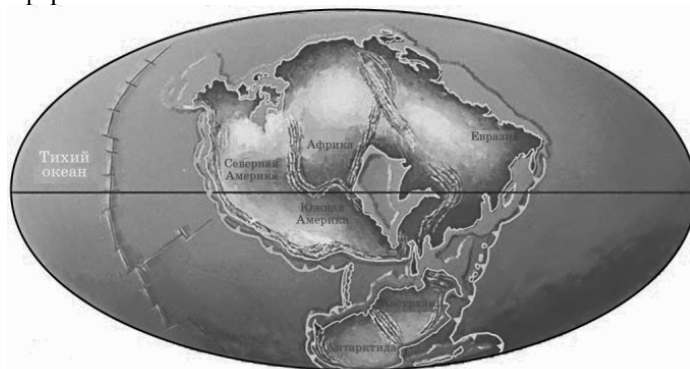
Рис. 2. Предполагаемое расположение континентов Пангеи Ультимы [Continents... 2000; см. также сайт: www.scotese.com ]
